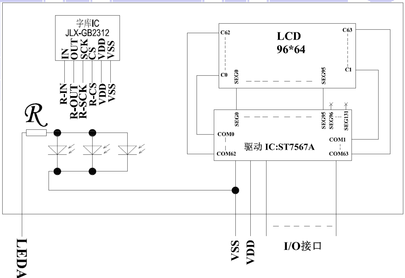
图 2: JLX9664G-958 图像点阵型液晶模块的电路框图
